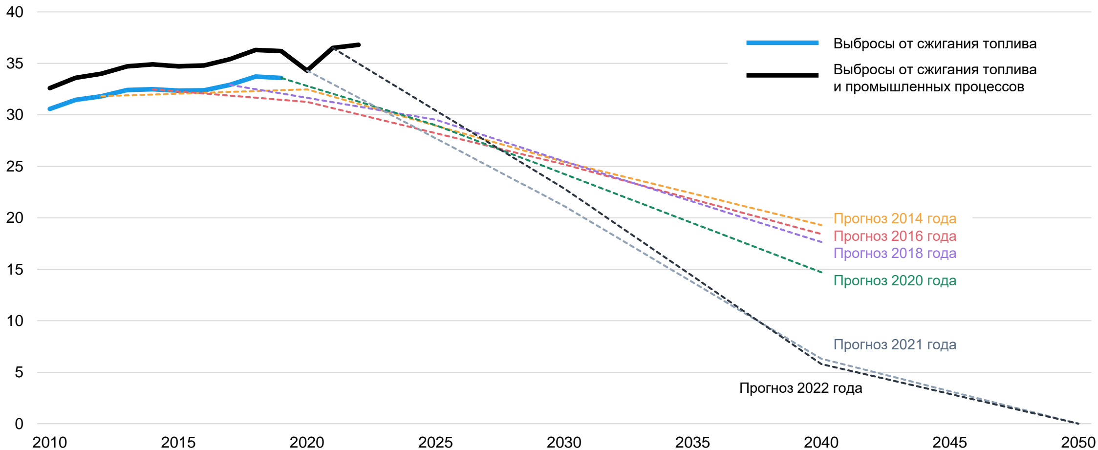
Выбросы CO 2 : реальность и амбициозные прогнозы (млрд т)
