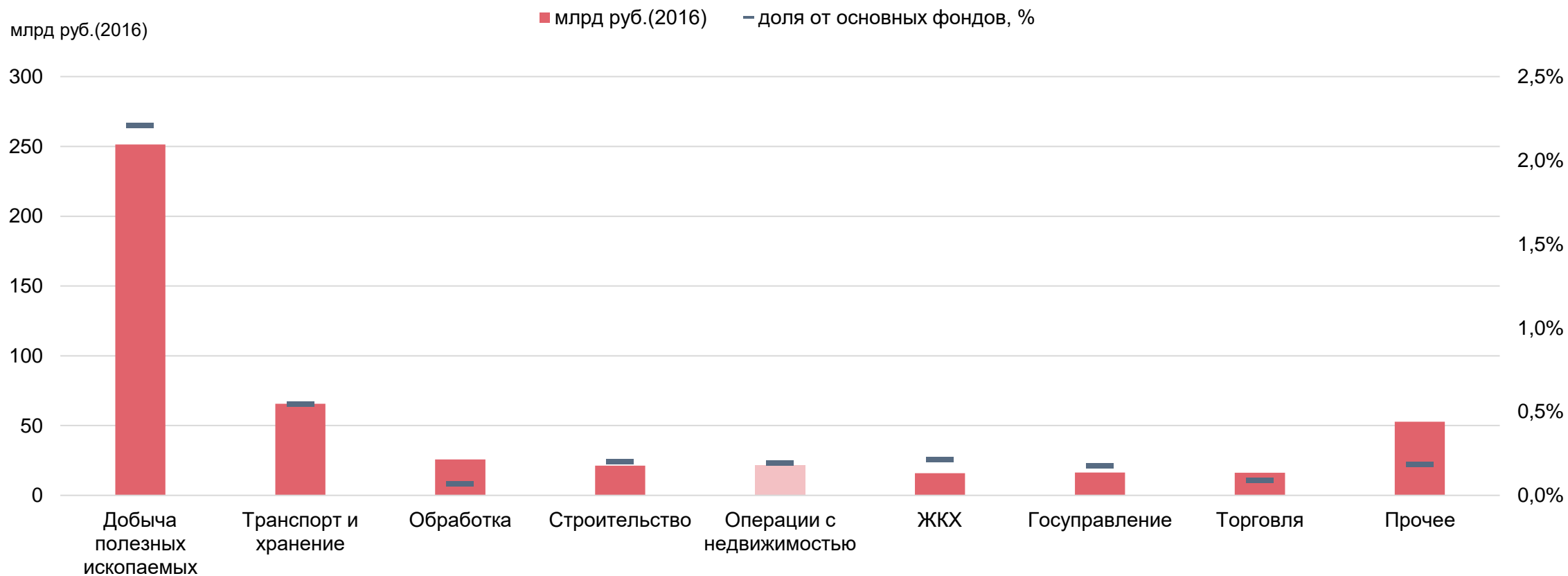
Потенциальный ущерб основным фондам от деградации многолетней мерзлоты в период до 2050 года
